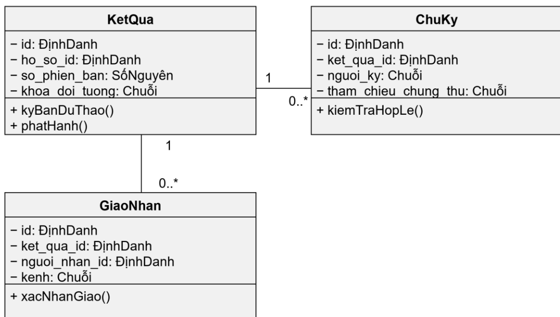
Biểu đồ lớp Chữ ký số
