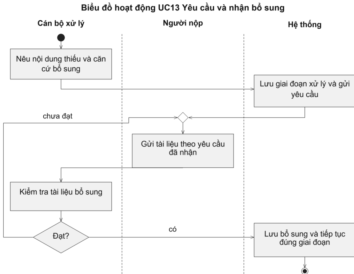
Hình 2.47: Biểu đồ hoạt động của Use case UC13
