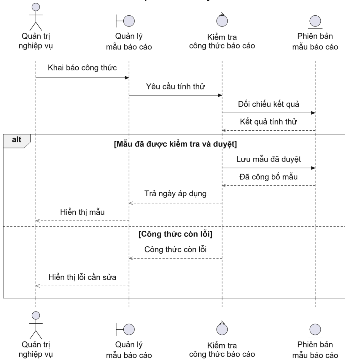
Hình 2.90: Biểu đồ trình tự của Use case UC24
