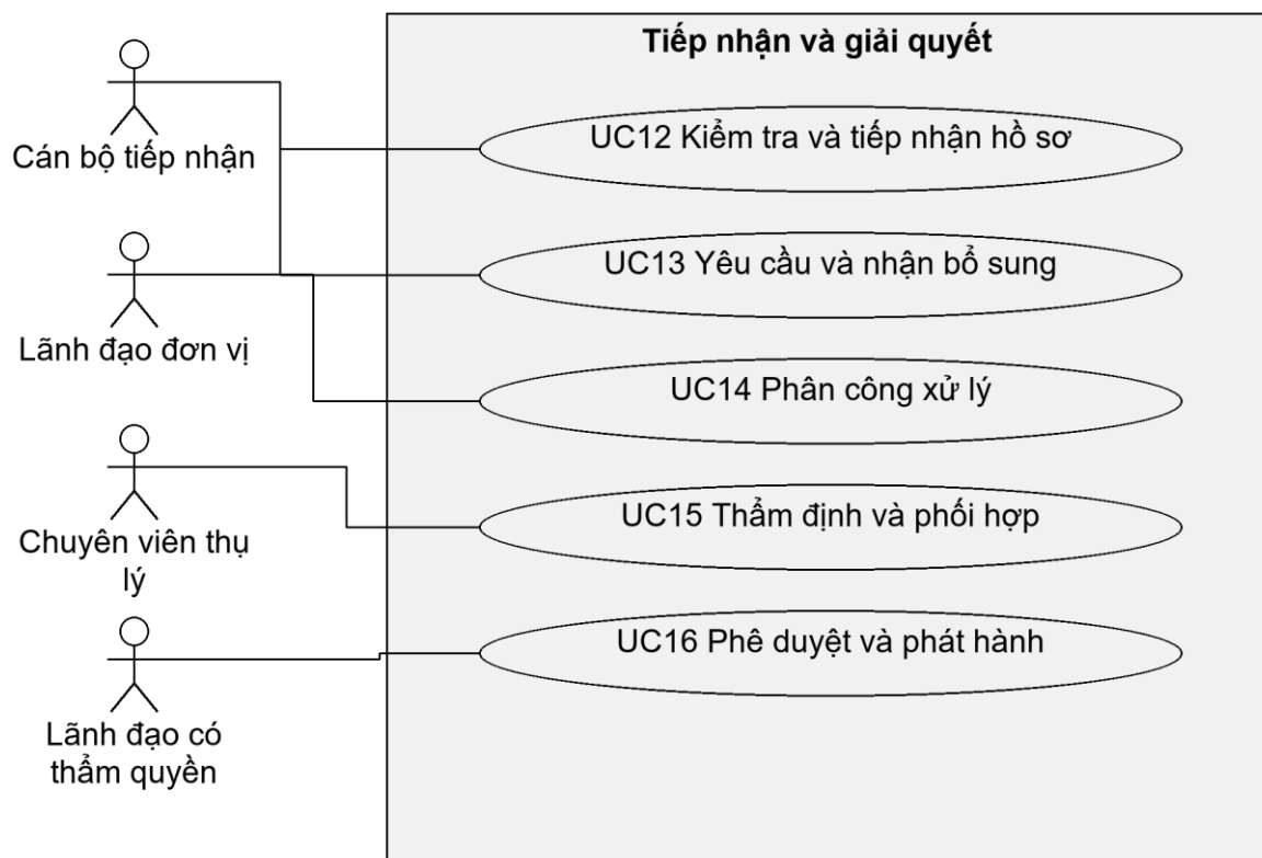
Hình 2.40: Use case nhóm 4, phần 1
