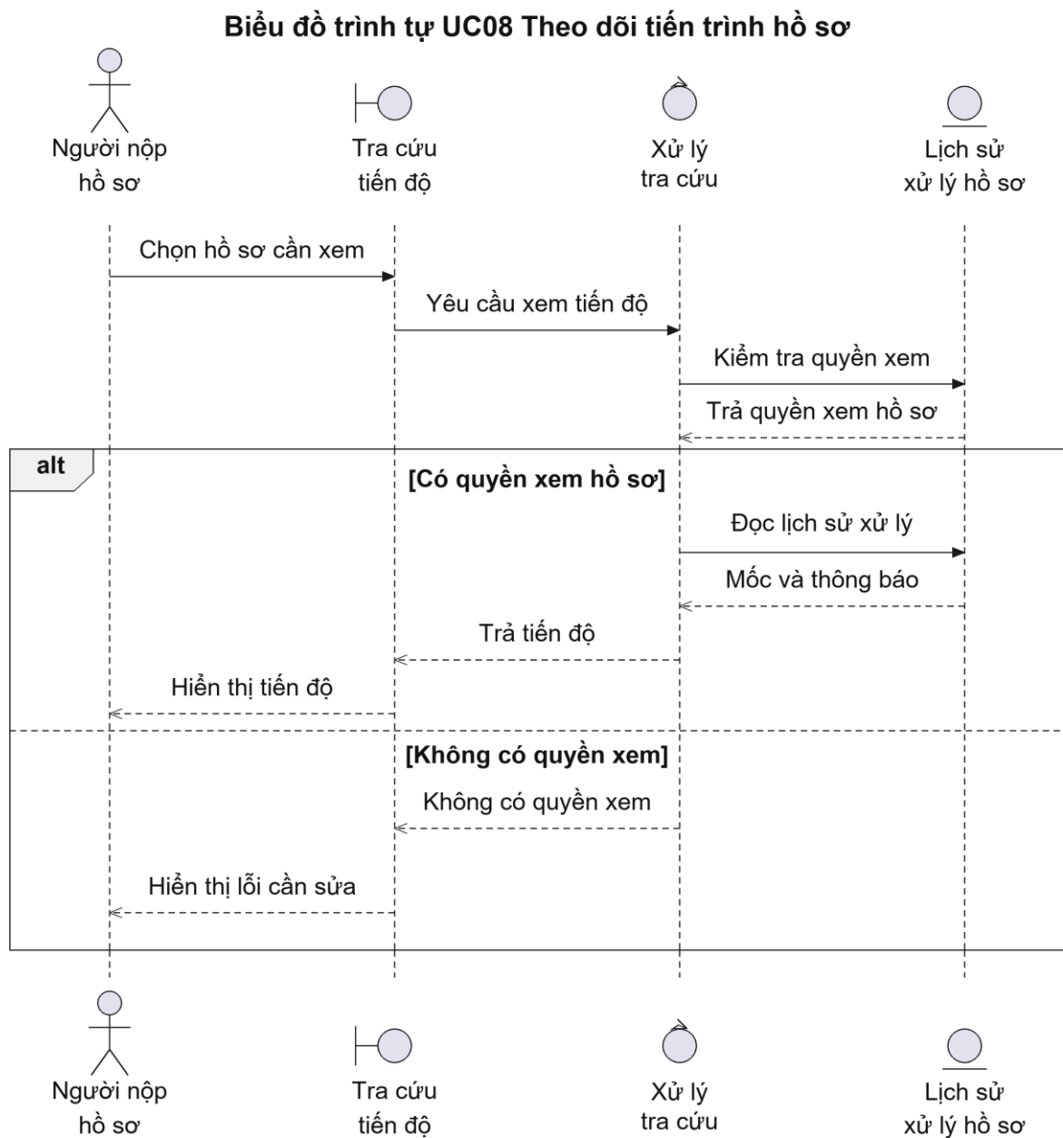
Hình 2.28: Biểu đồ trình tự của Use case UC08
