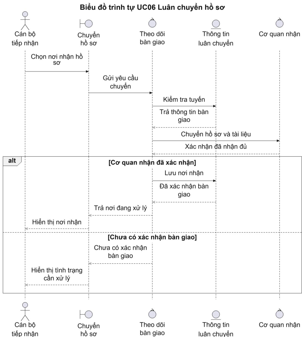
Hình 2.22: Biểu đồ trình tự của Use case UC06
