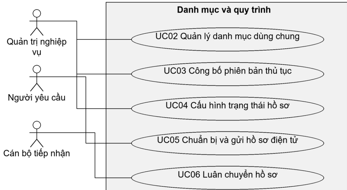
Hình 2.7: Use case nhóm 2, phần 1
