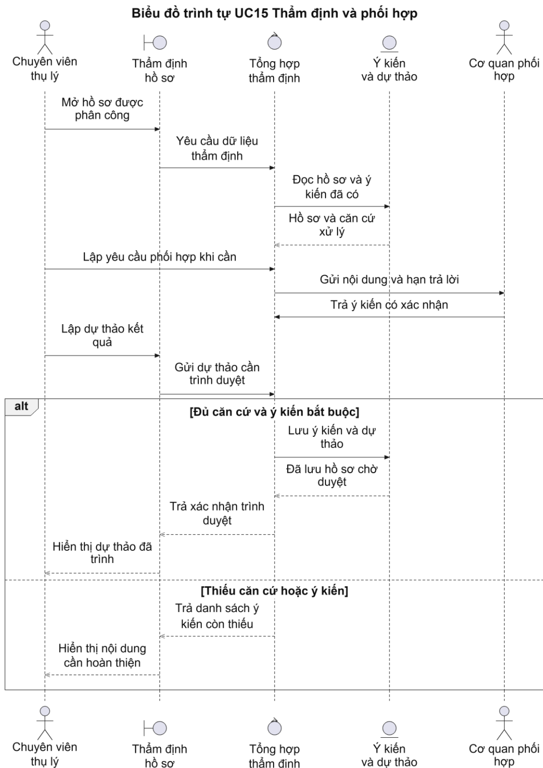
Hình 2.52: Biểu đồ trình tự của Use case UC15
