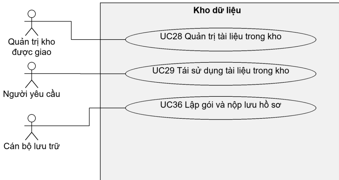
Hình 2.105: Use case nhóm 8
