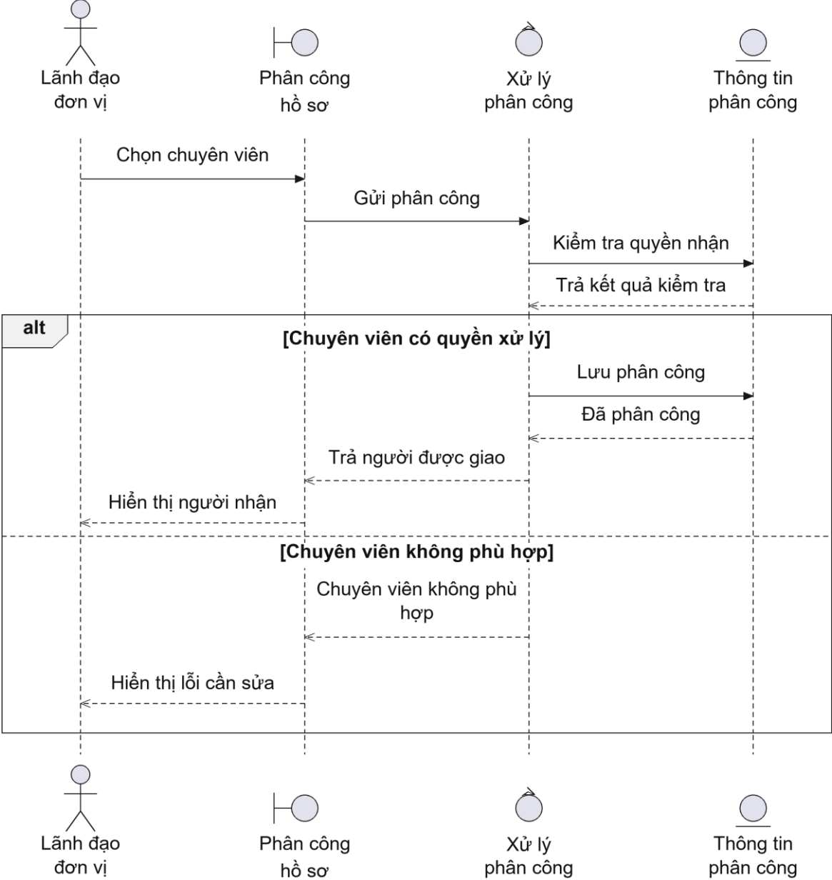
Biểu đồ trình tự UC14 Phân công xử lý
