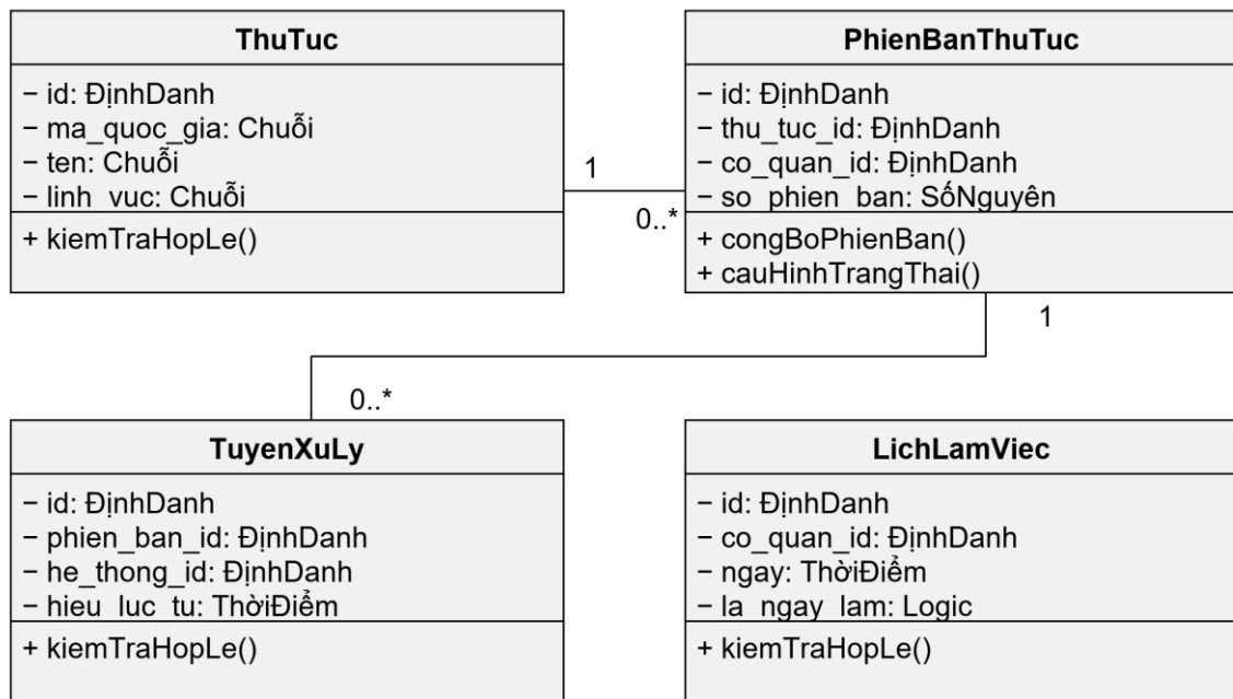
Biểu đồ lớp Danh mục và quy trình
