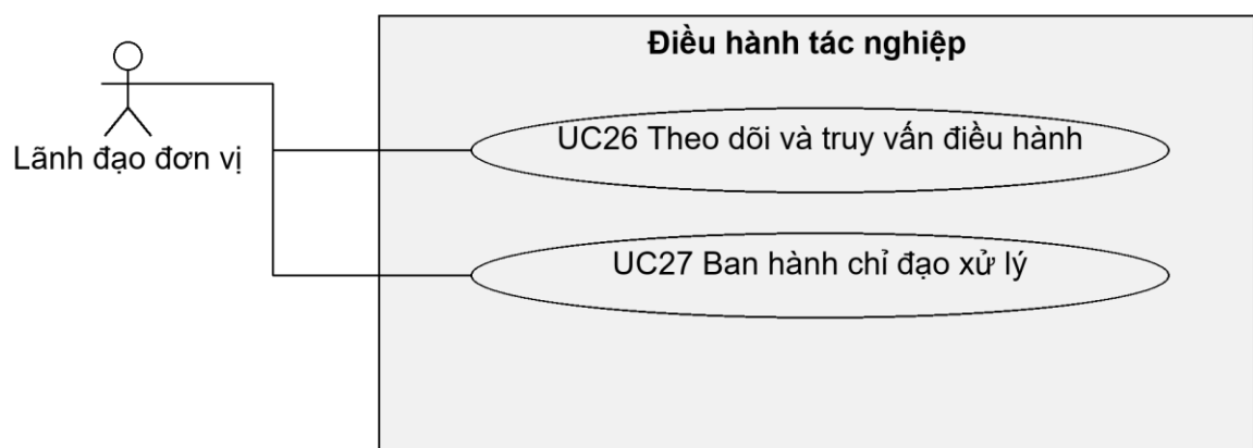
Hình 2.98: Use case nhóm 7
