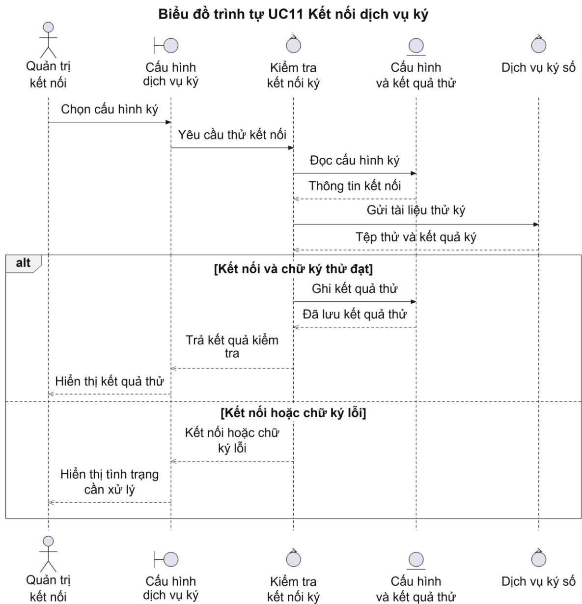
Hình 2.38: Biểu đồ trình tự của Use case UC11
