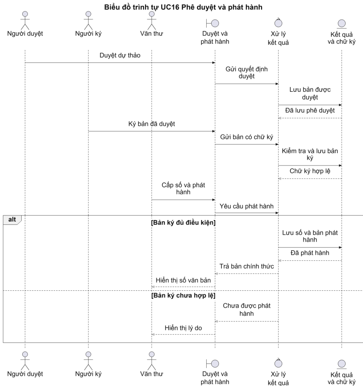
Hình 2.55: Biểu đồ trình tự của Use case UC16
