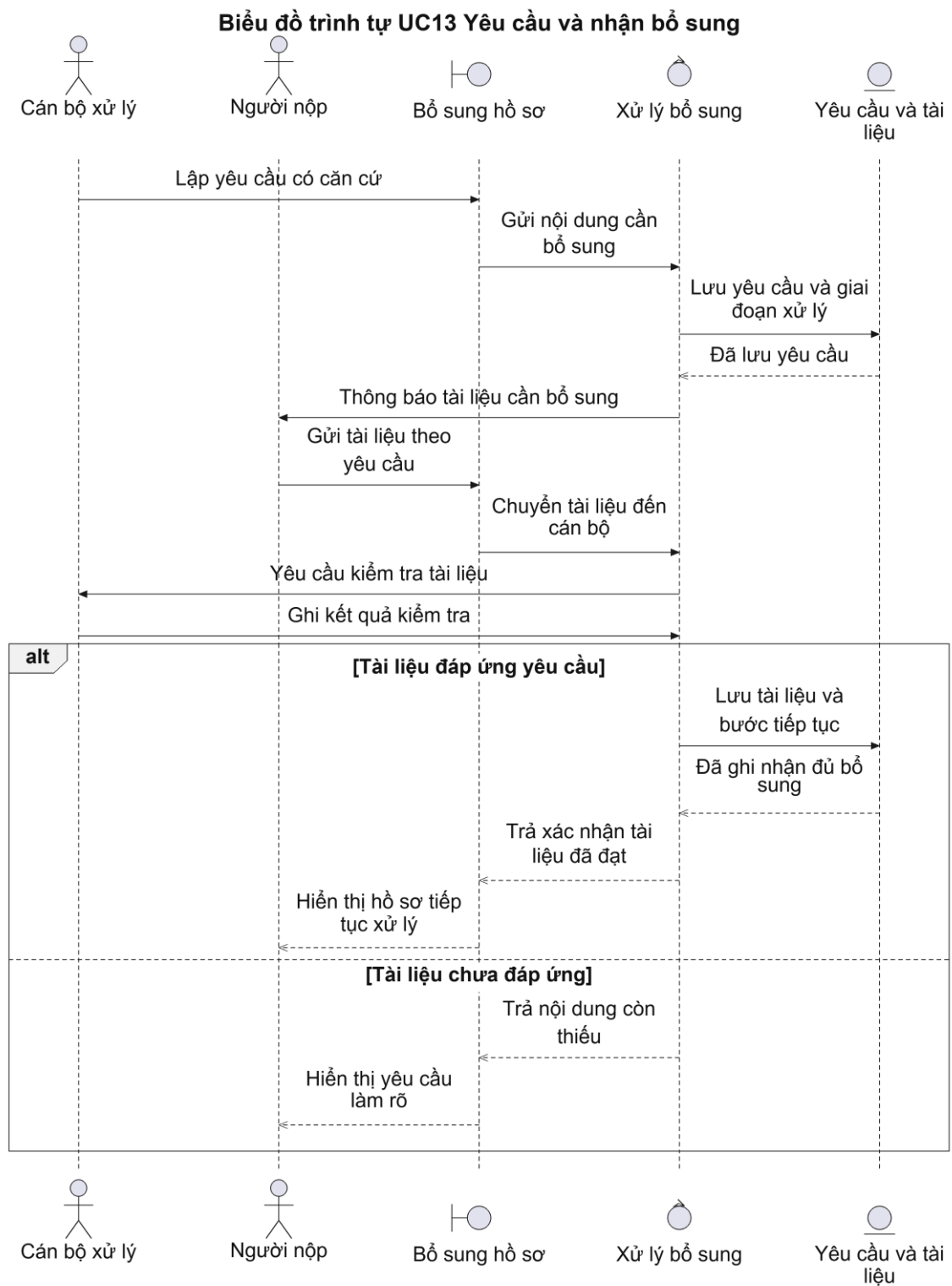
Hình 2.46: Biểu đồ trình tự của Use case UC13
