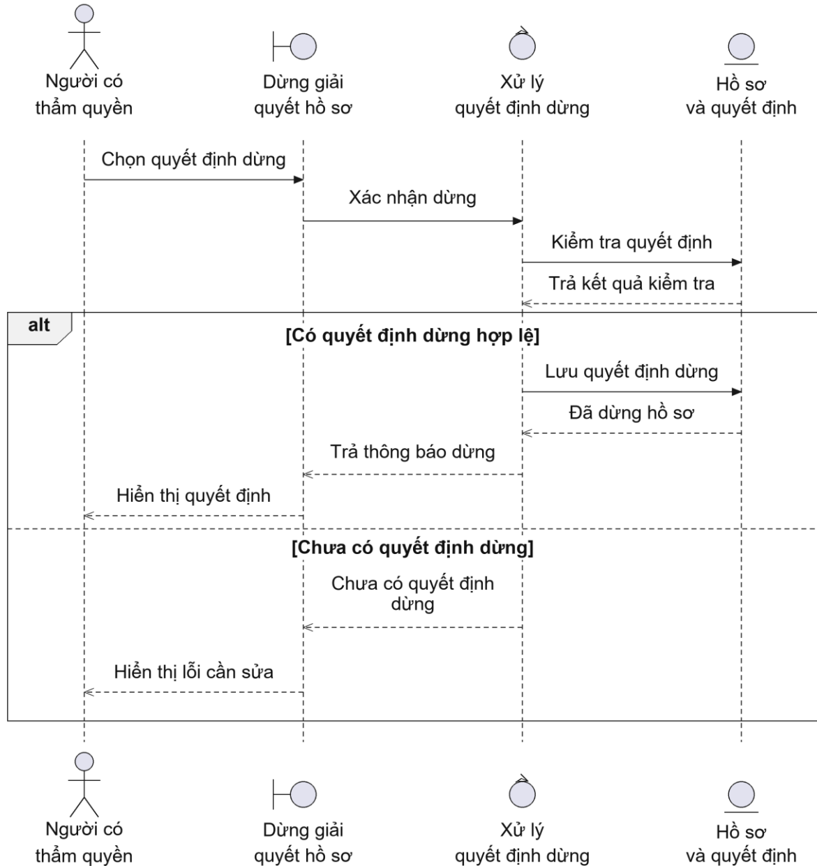
Hình 2.58: Biểu đồ trình tự của Use case UC17
