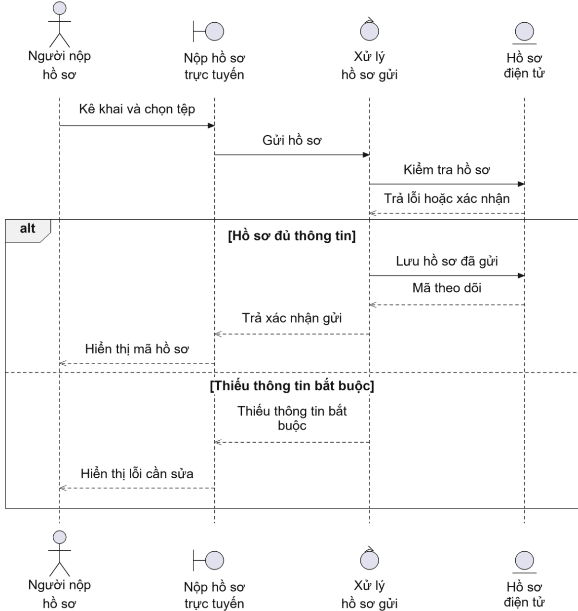
Hình 2.19: Biểu đồ trình tự của Use case UC05
