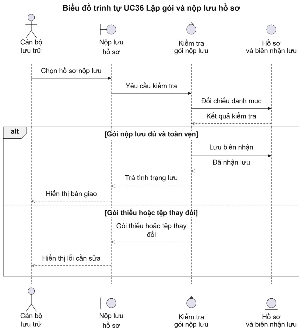
Hình 2.113: Biểu đồ trình tự của Use case UC36
