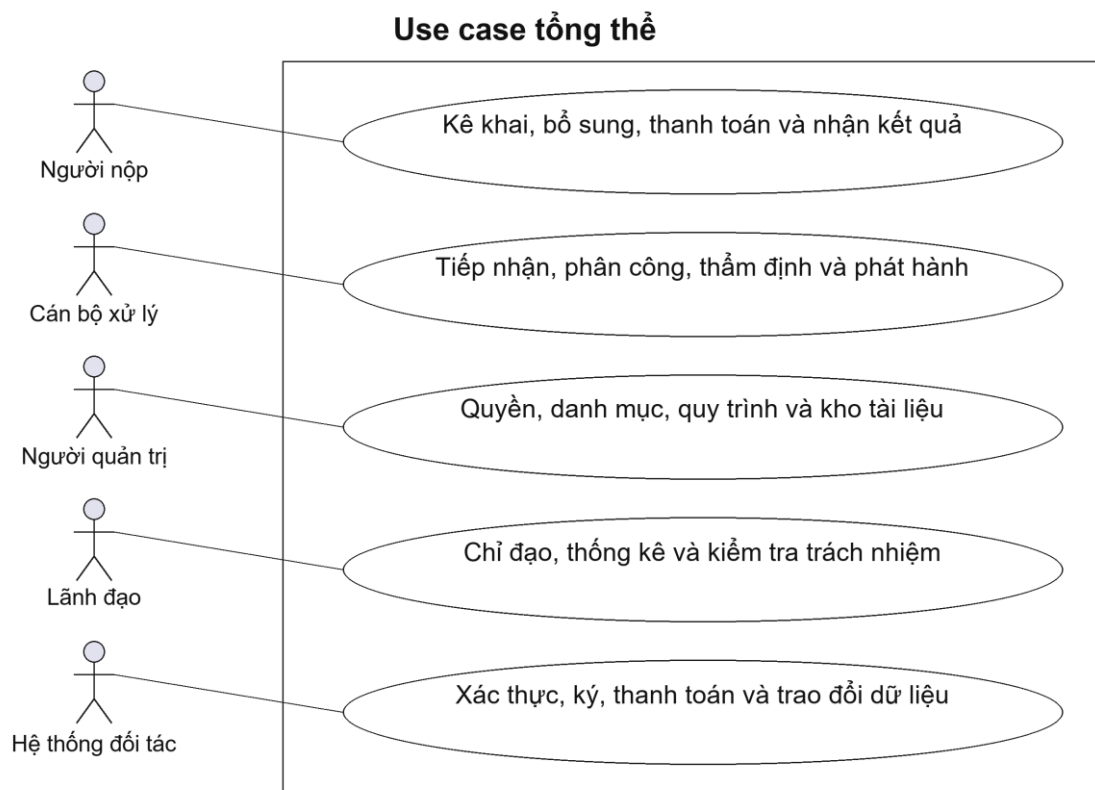
Hình 2.2: Use case tổng thể theo mục tiêu
