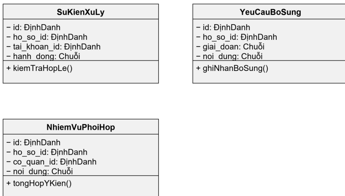
Biểu đồ lớp Tiếp nhận và giải quyết phần 2
