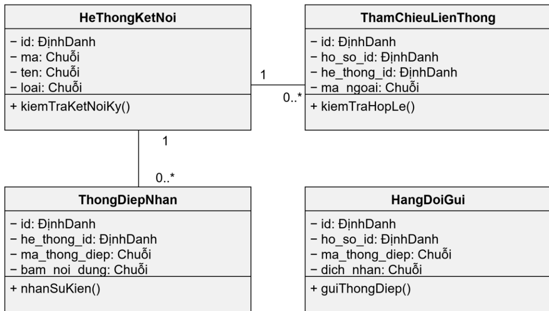
Biểu đồ lớp Tích hợp và liên thông
