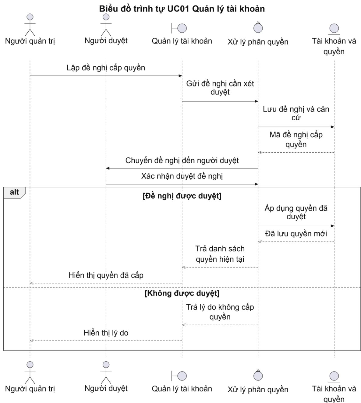
Hình 2.5: Biểu đồ trình tự của Use case UC01
