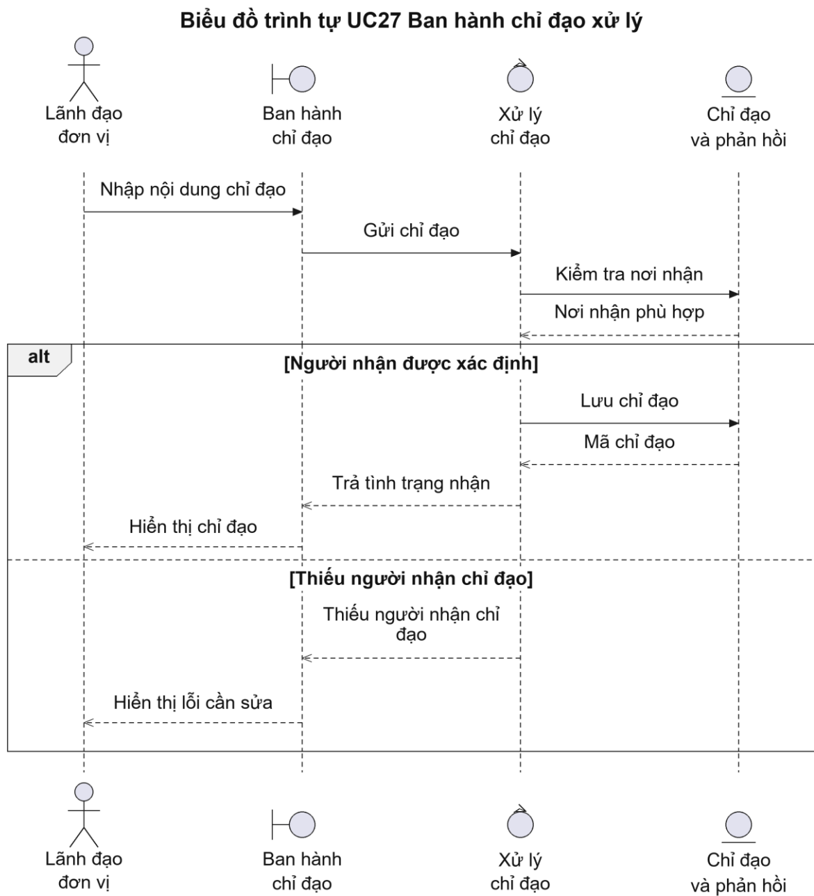
Hình 2.103: Biểu đồ trình tự của Use case UC27
