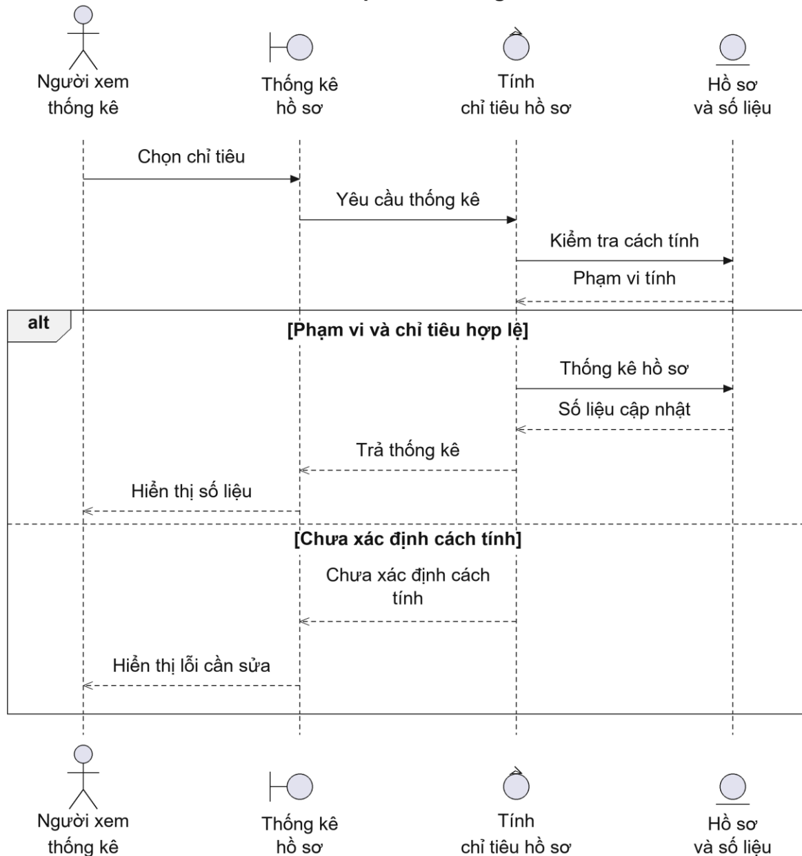
Hình 2.93: Biểu đồ trình tự của Use case UC25
