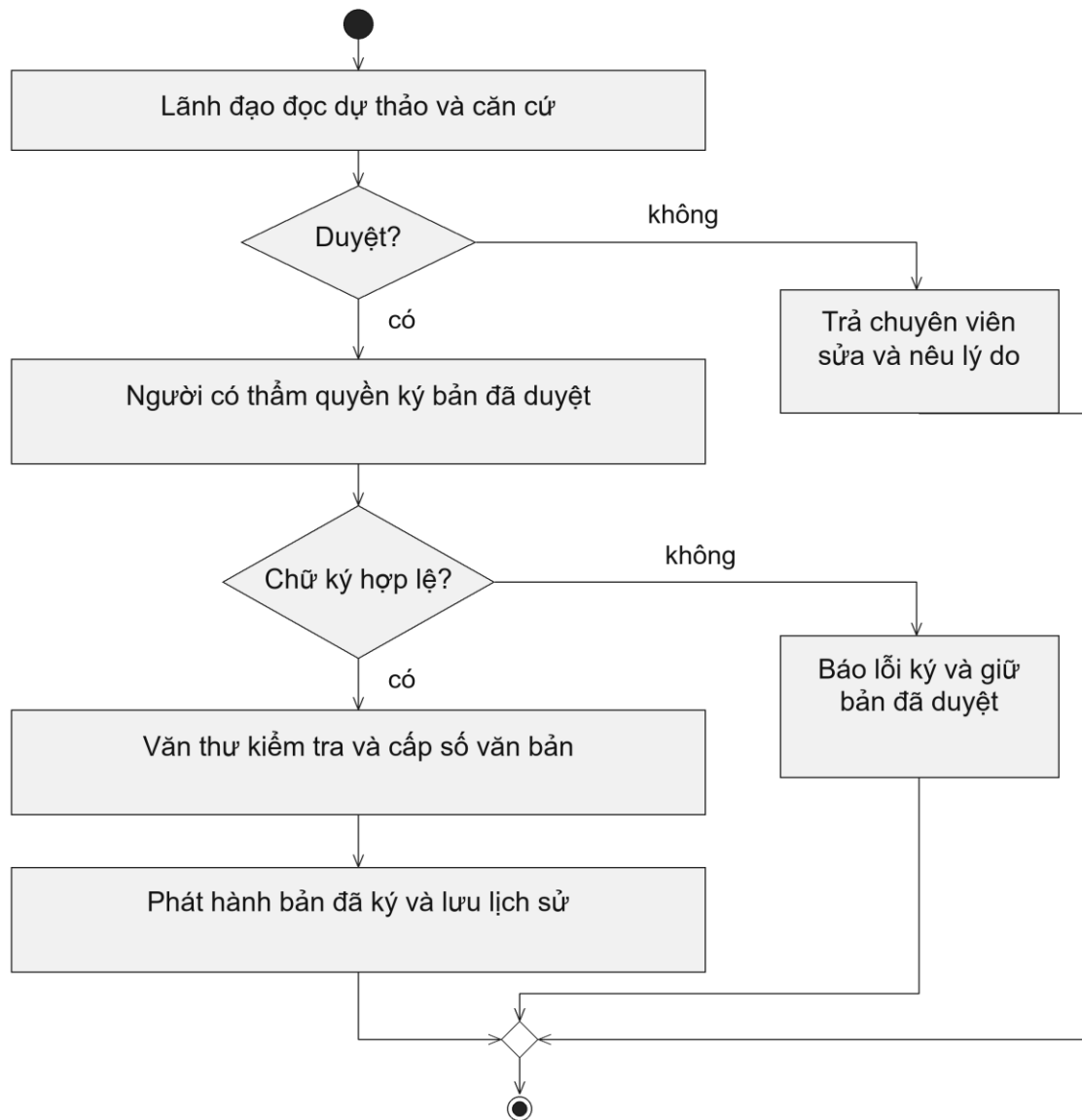
Biểu đồ hoạt động UC16 Phê duyệt và phát hành
