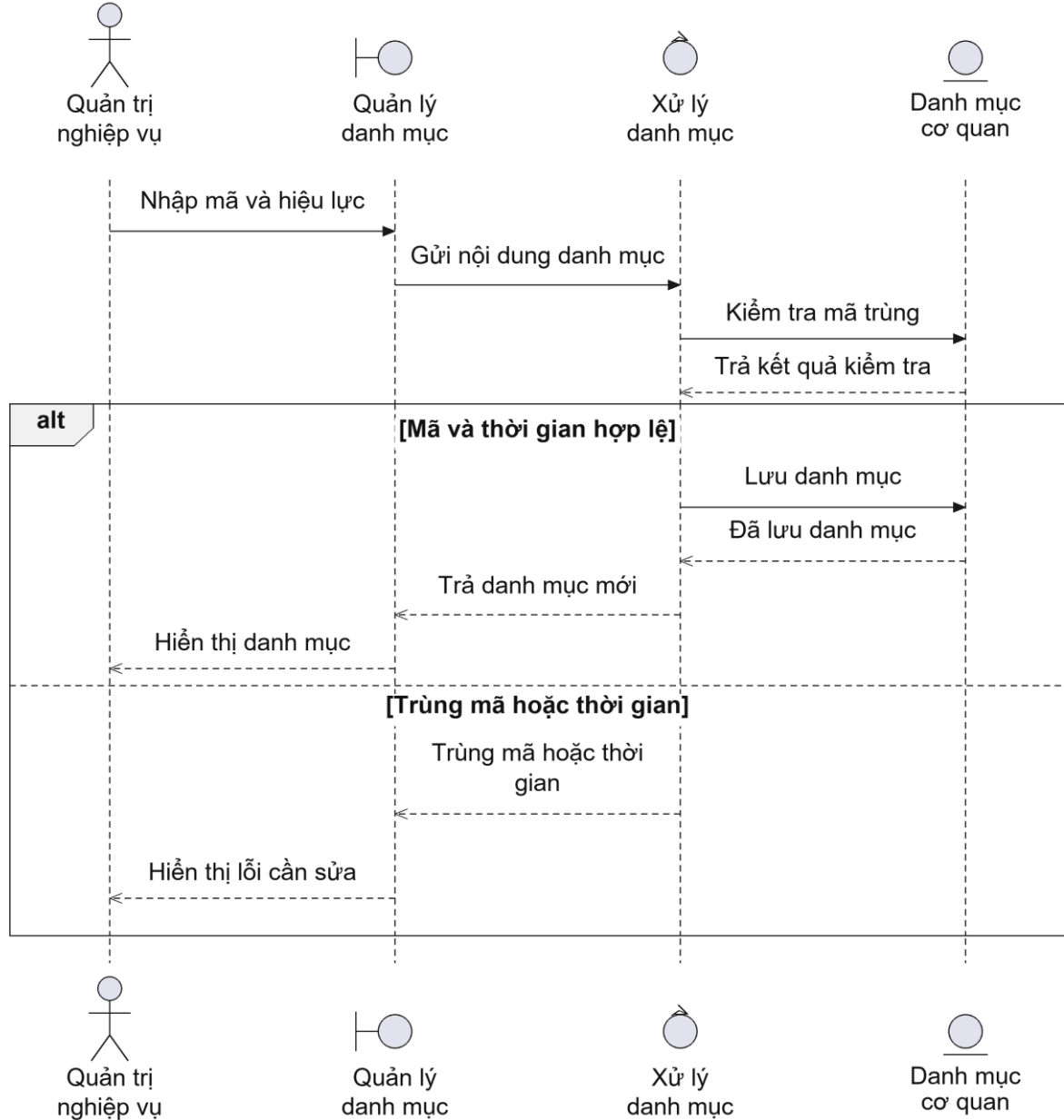
Hình 2.10: Biểu đồ trình tự của Use case UC02
