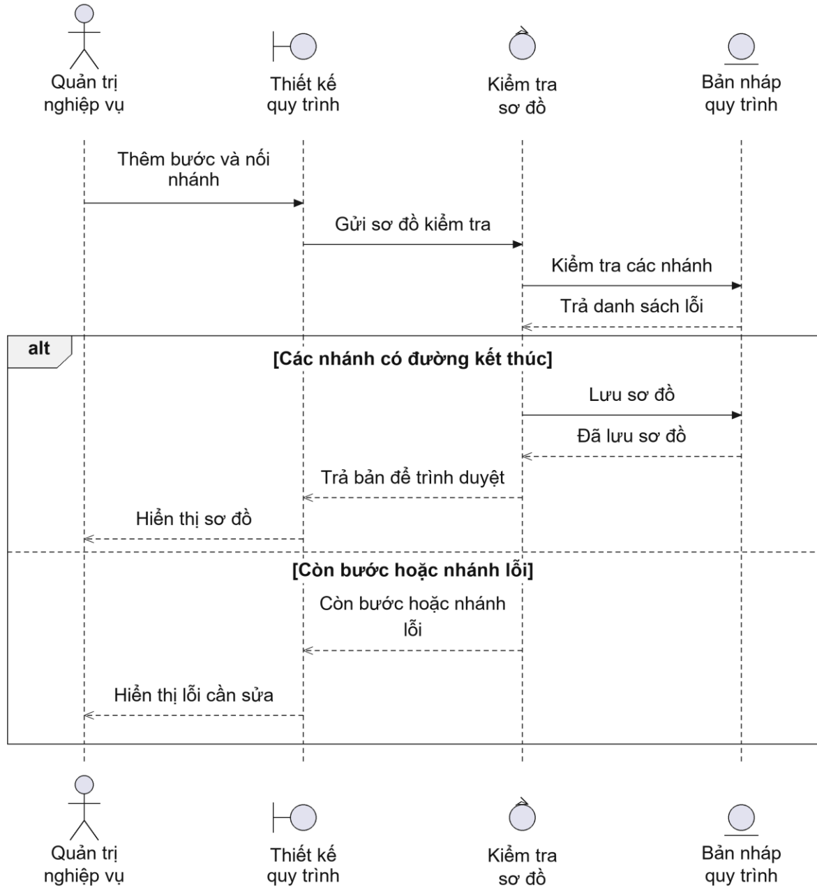
Hình 2.31: Biểu đồ trình tự của Use case UC09
