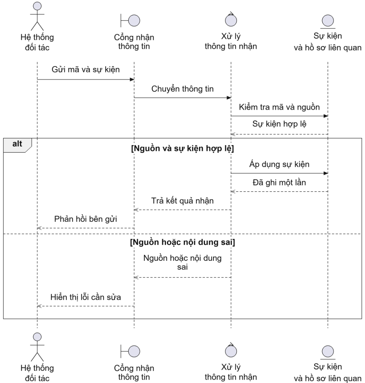
Hình 2.117: Biểu đồ trình tự của Use case UC30
