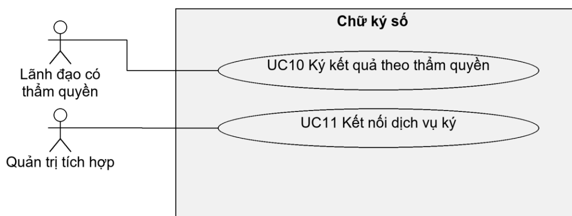
Hình 2.33: Use case nhóm 3
