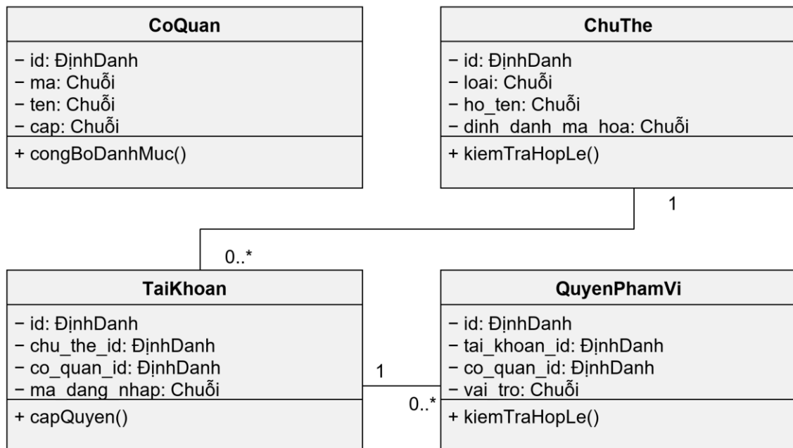
Biểu đồ lớp Tài khoản và quyền
