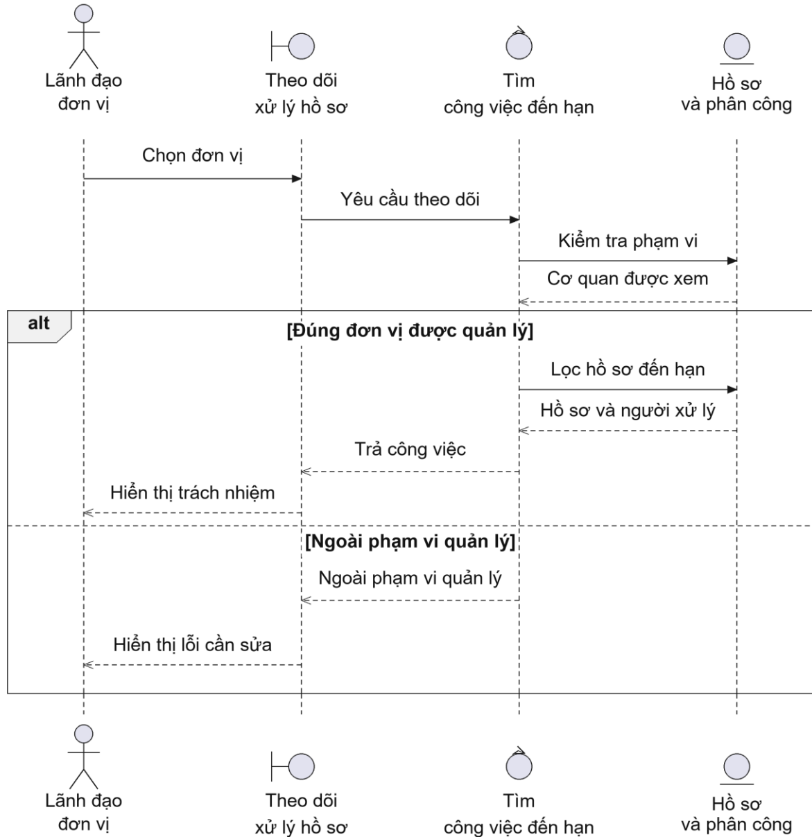
Hình 2.100: Biểu đồ trình tự của Use case UC26
