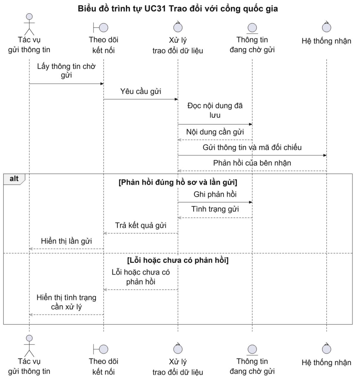
Hình 2.120: Biểu đồ trình tự của Use case UC31
