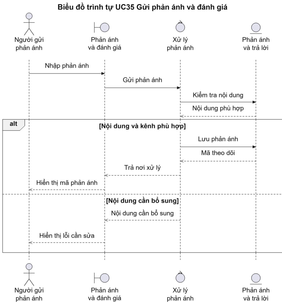
Hình 2.83: Biểu đồ trình tự của Use case UC35
