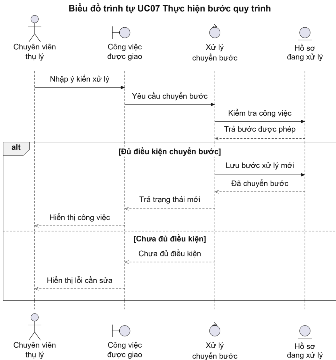
Hình 2.25: Biểu đồ trình tự của Use case UC07
