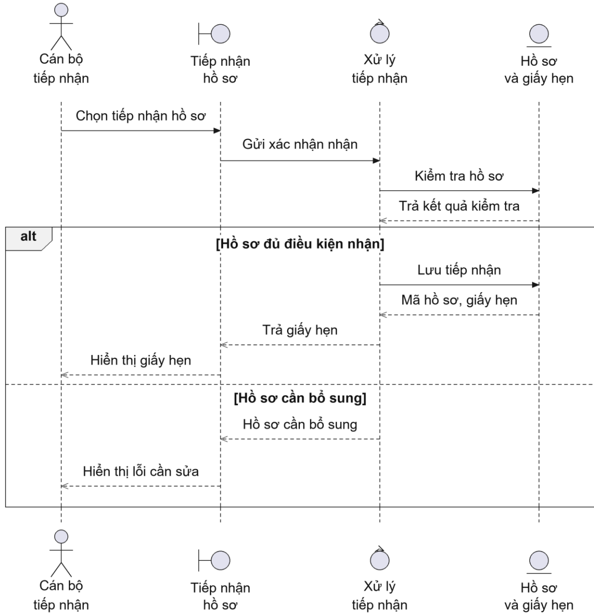
Hình 2.43: Biểu đồ trình tự của Use case UC12
