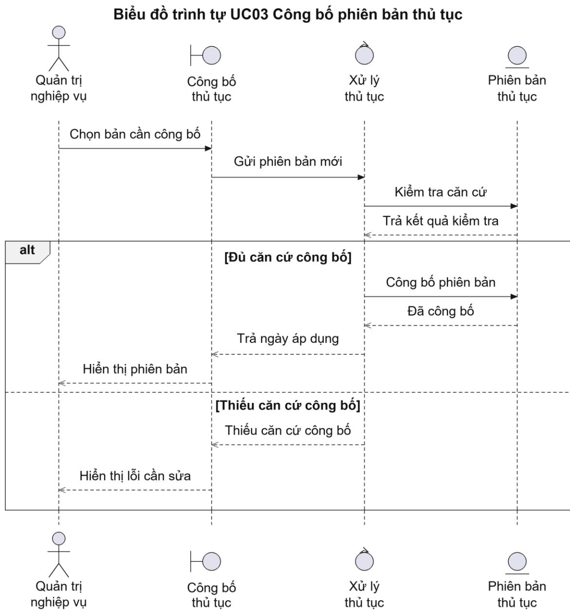
Hình 2.13: Biểu đồ trình tự của Use case UC03
