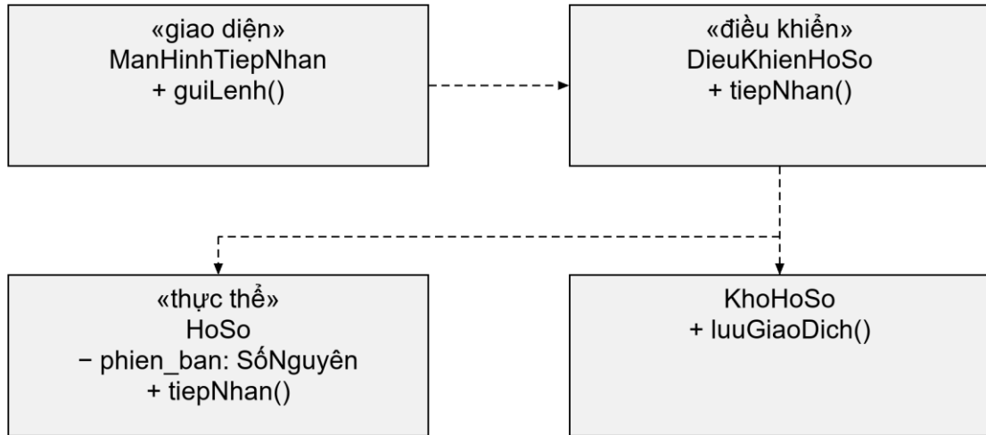
Lớp phân tích của Use case tiếp nhận
