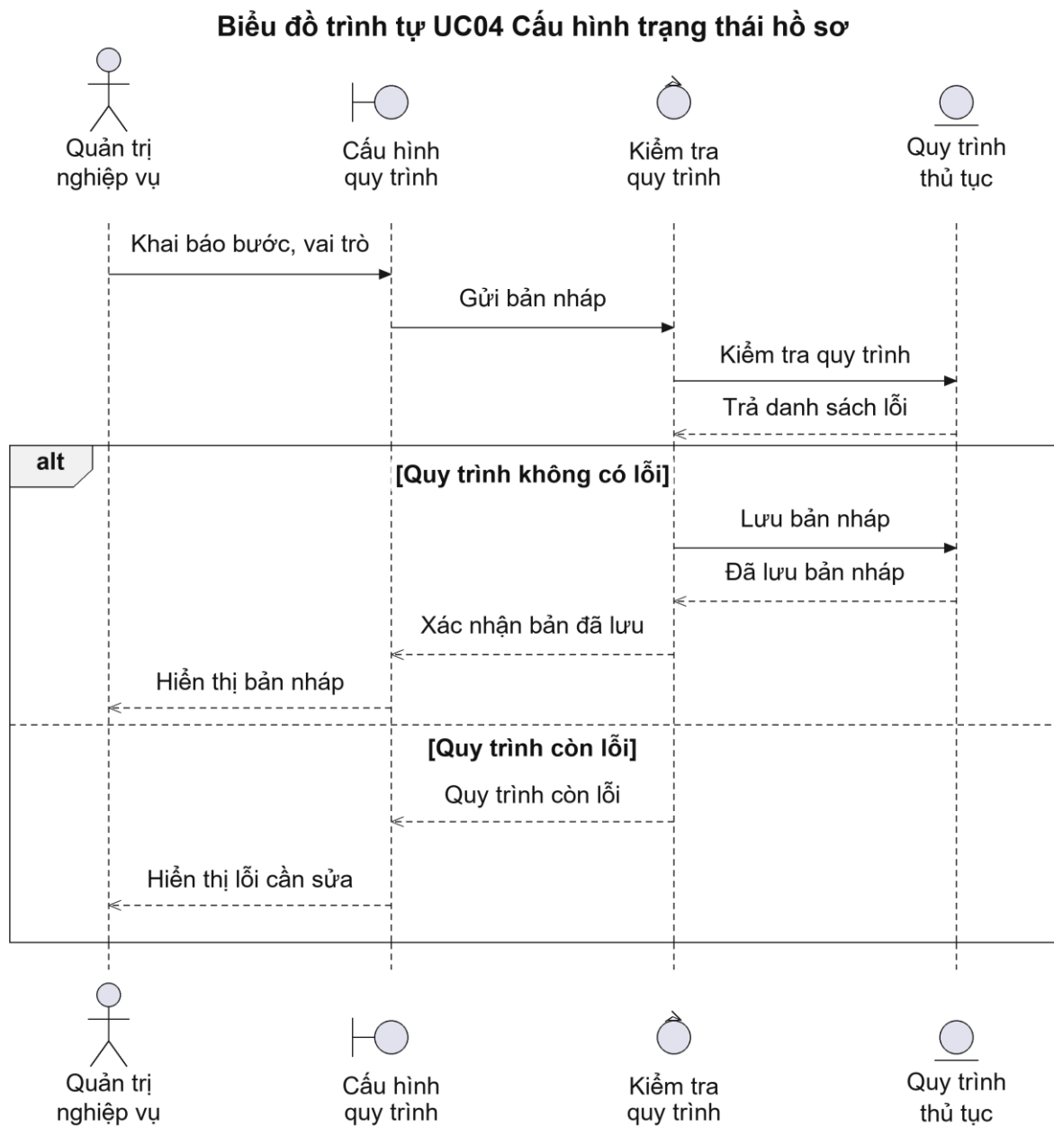
Hình 2.16: Biểu đồ trình tự của Use case UC04
