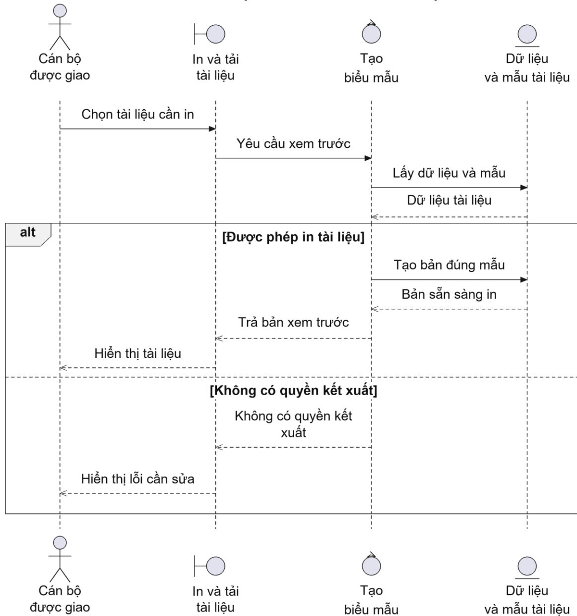
Hình 2.71: Biểu đồ trình tự của Use case UC19
