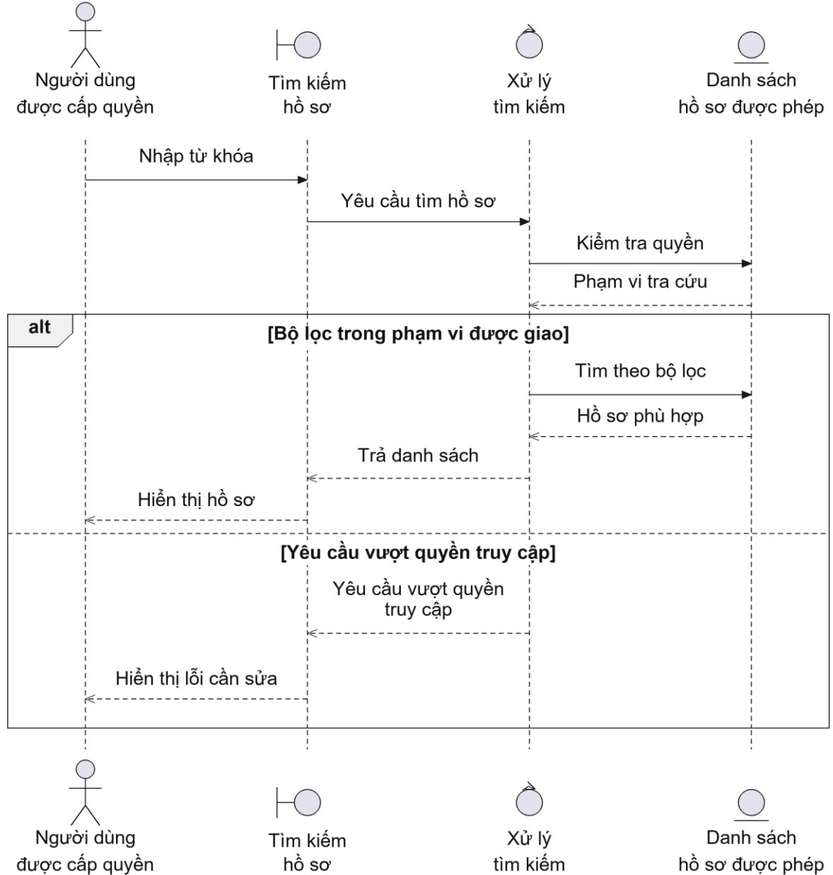
Hình 2.77: Biểu đồ trình tự của Use case UC21
