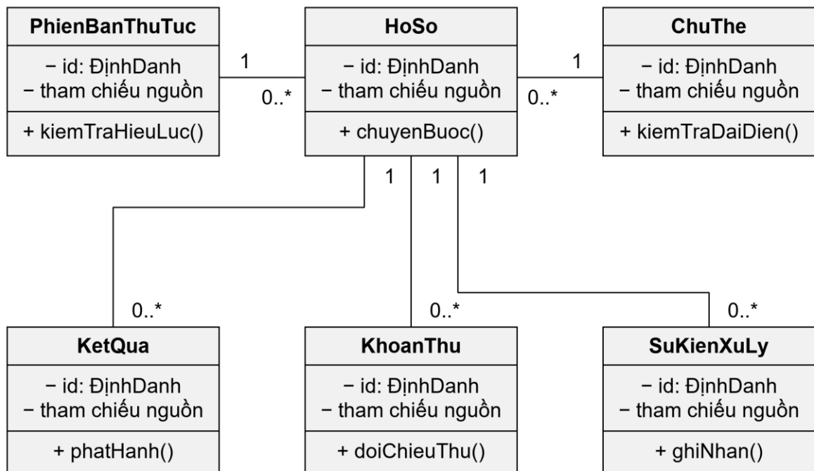
Quan hệ miền cốt lõi quanh hồ sơ
