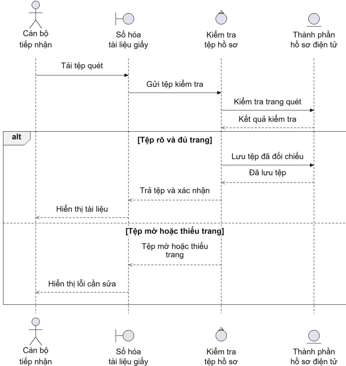
Hình 2.67: Biểu đồ trình tự của Use case UC34
