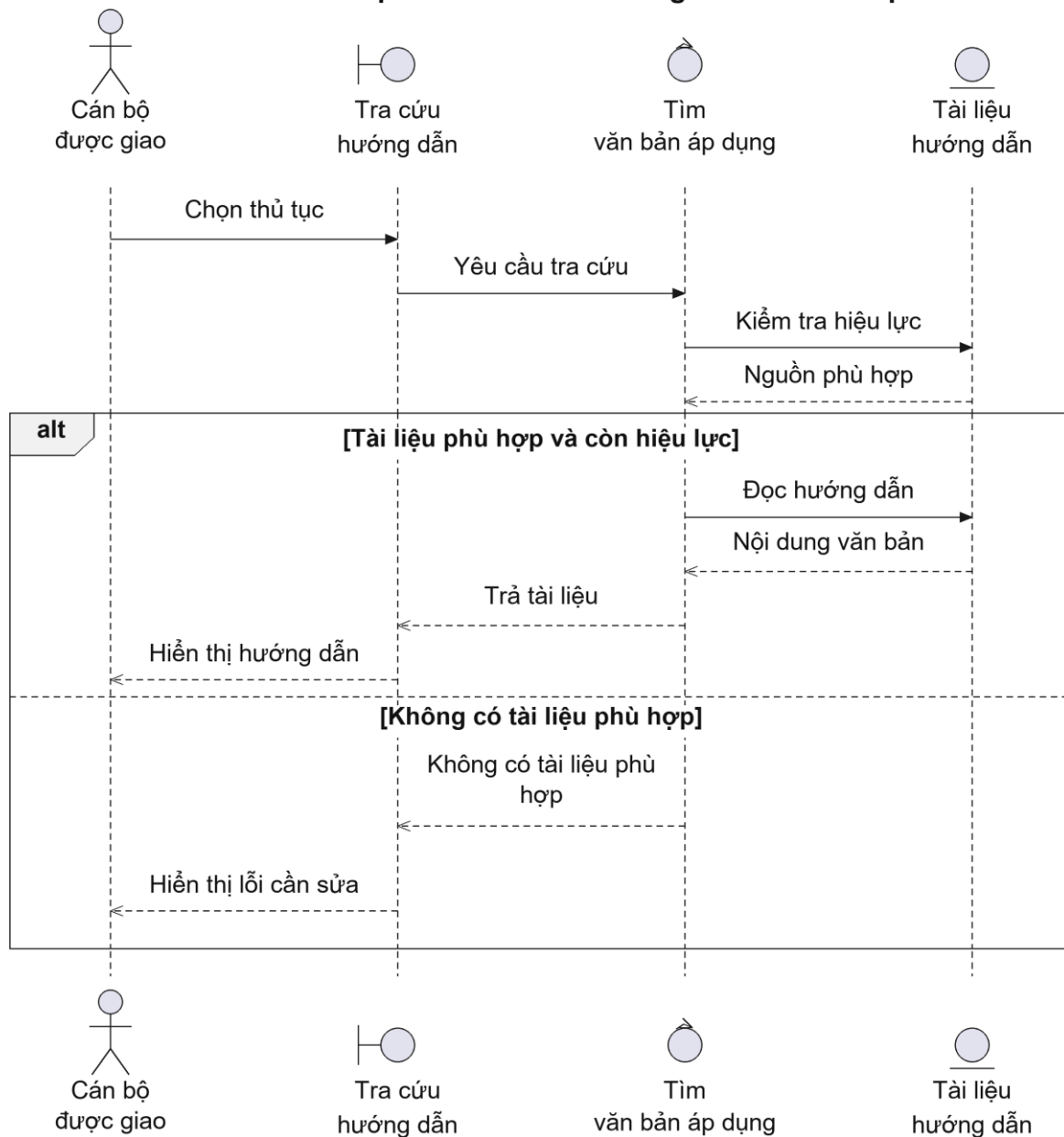
Hình 2.80: Biểu đồ trình tự của Use case UC22
