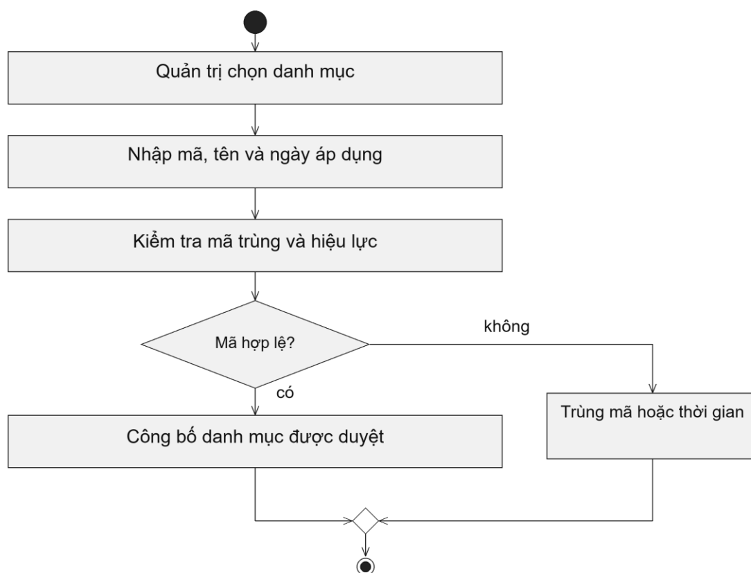
Biểu đồ hoạt động UC02 Quản lý danh mục dùng chung
