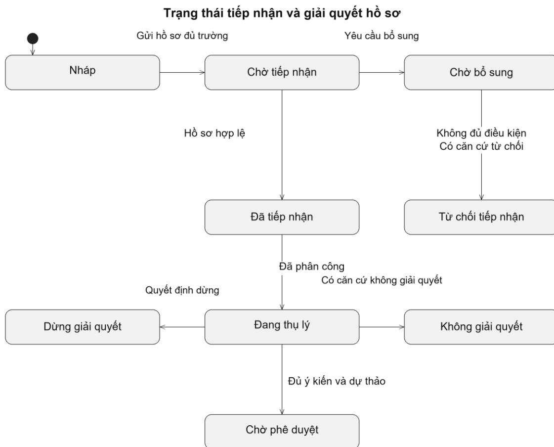
Hình 3.13: Các nhánh tiếp nhận và kết luận
