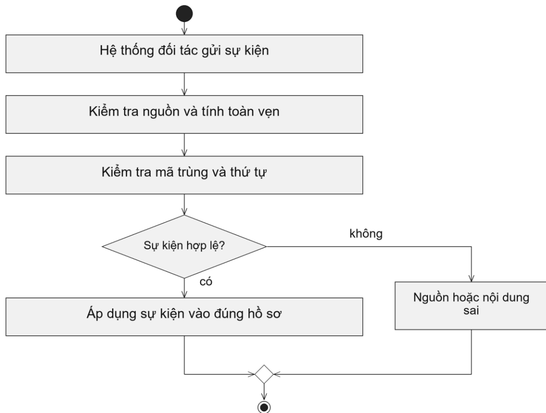
Biểu đồ hoạt động UC30 Nhận sự kiện từ hệ thống kết nối
