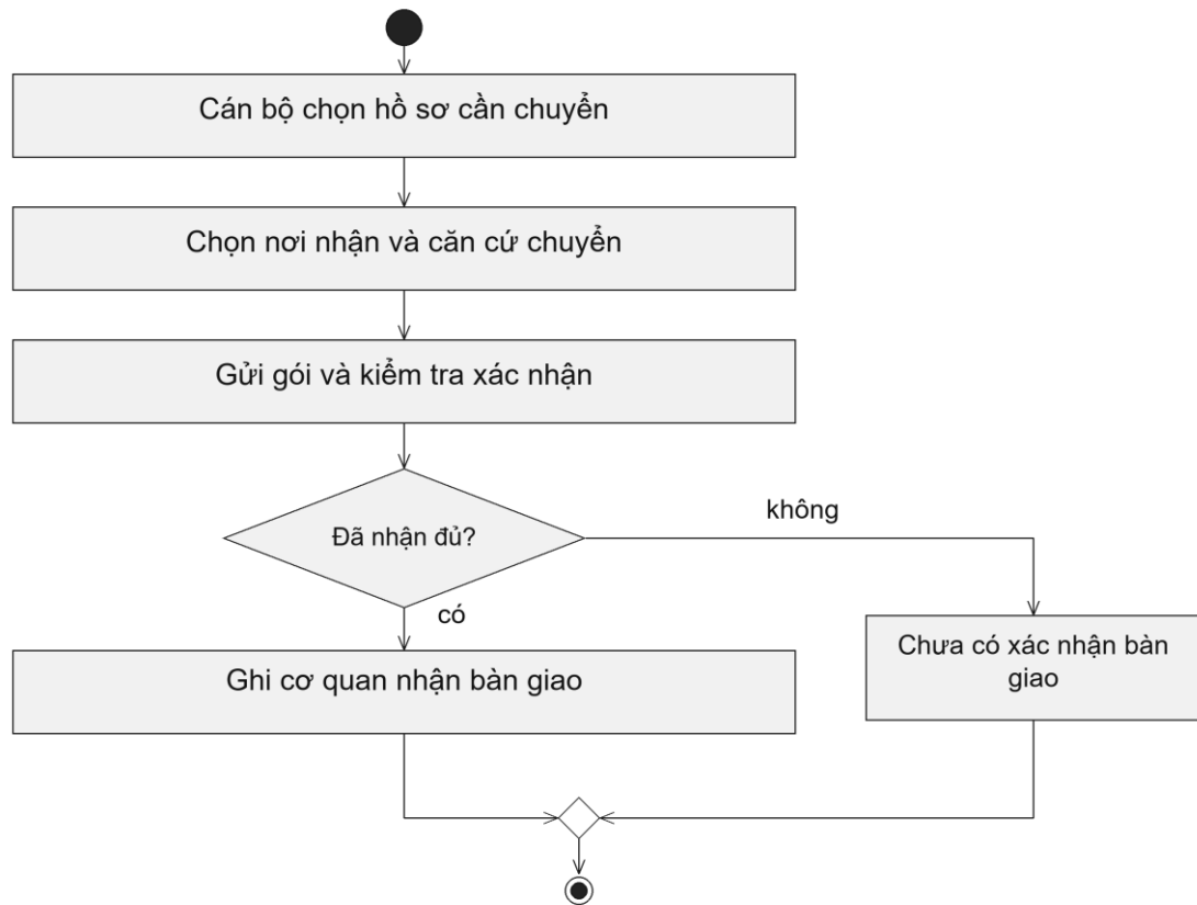
Biểu đồ hoạt động UC06 Luân chuyển hồ sơ
