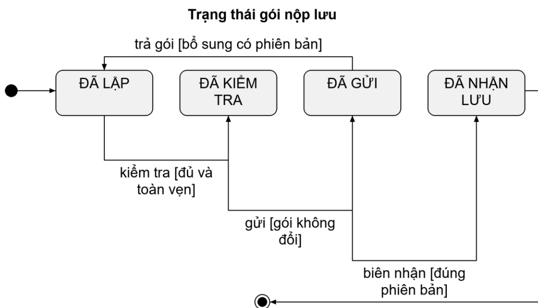
Hình 3.20: Vòng đời gói nộp lưu
