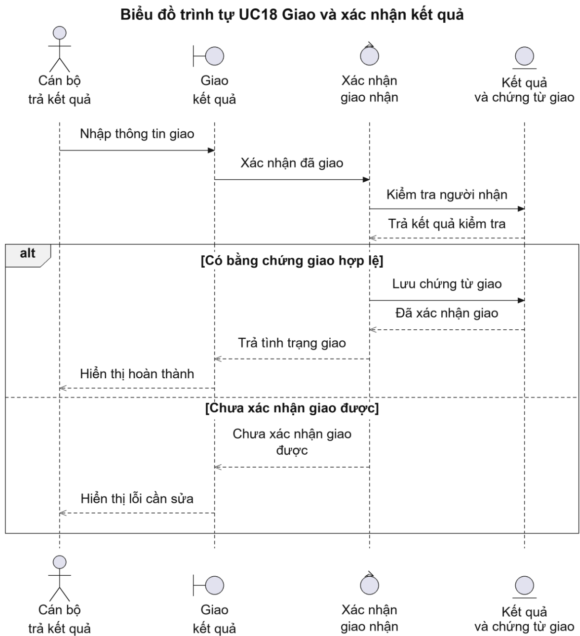
Hình 2.61: Biểu đồ trình tự của Use case UC18
