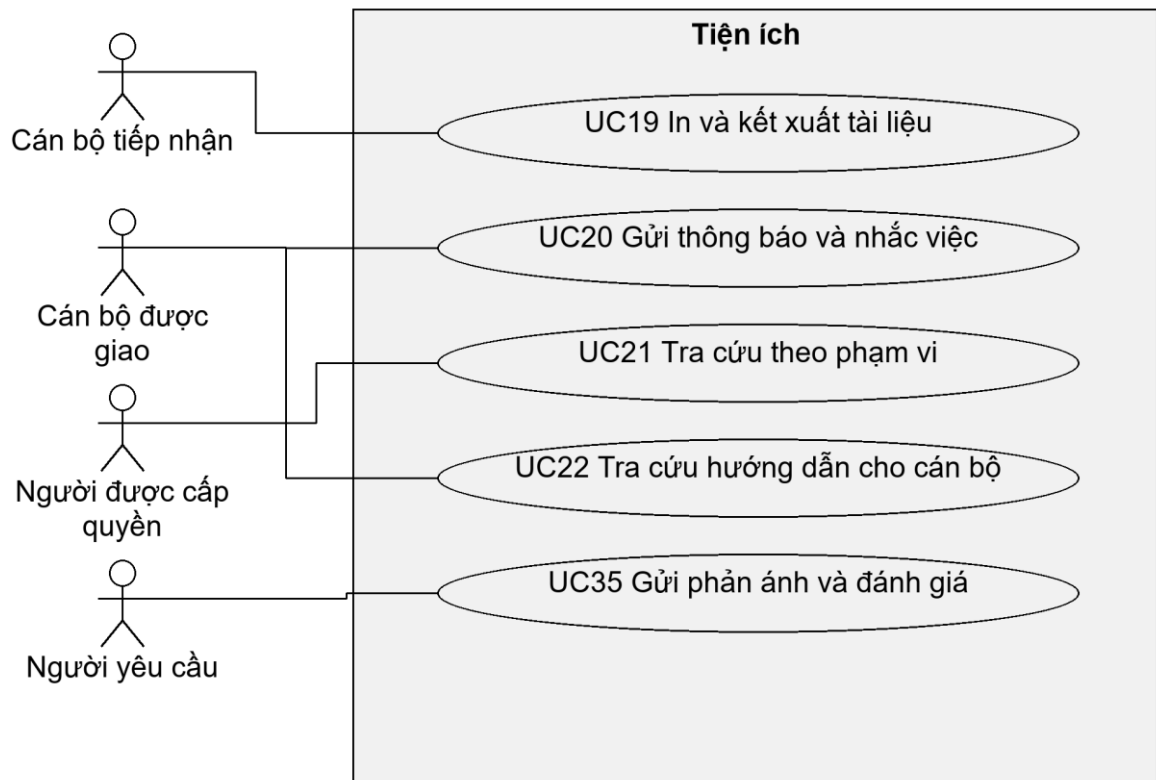
Hình 2.69: Use case nhóm 5
