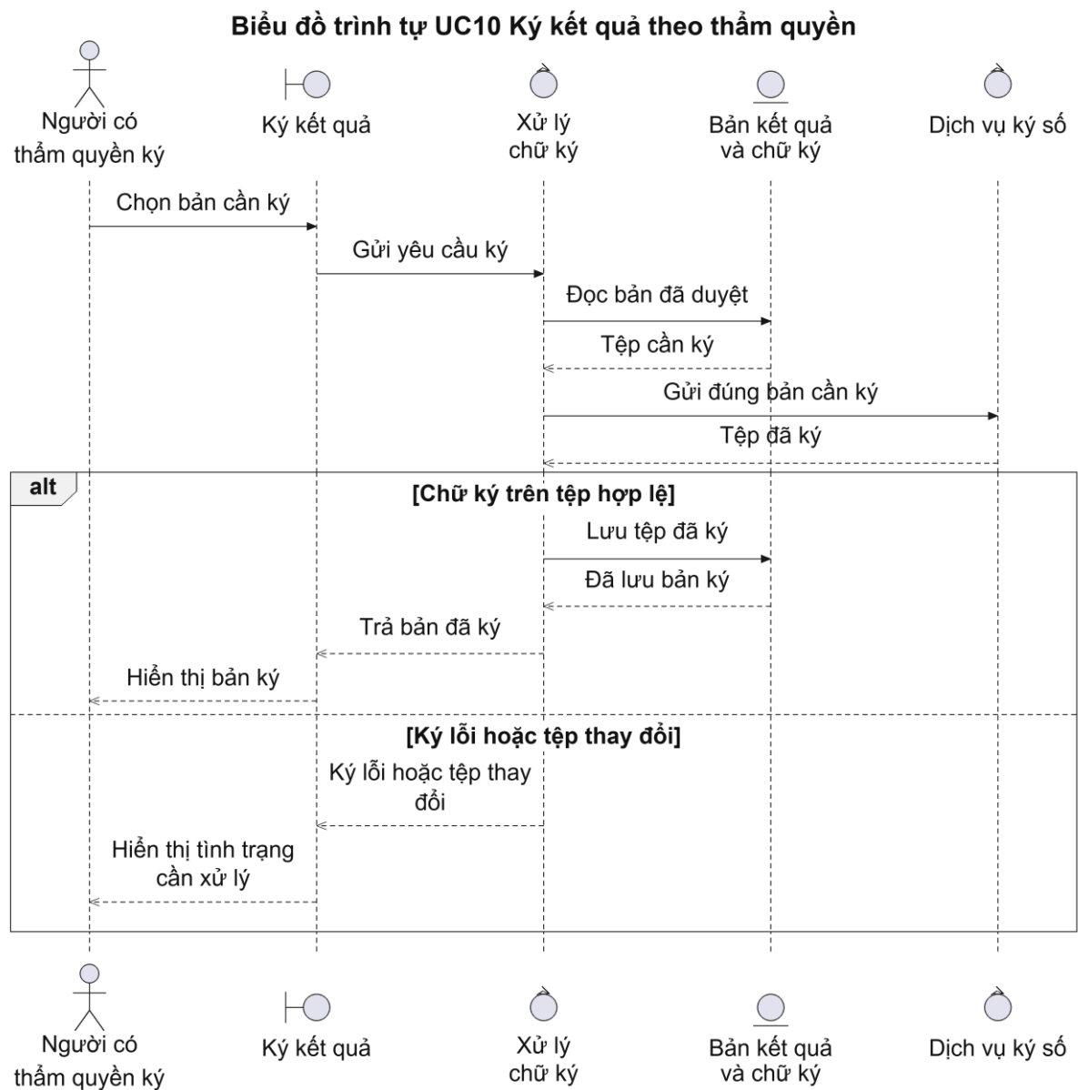
Hình 2.35: Biểu đồ trình tự của Use case UC10
