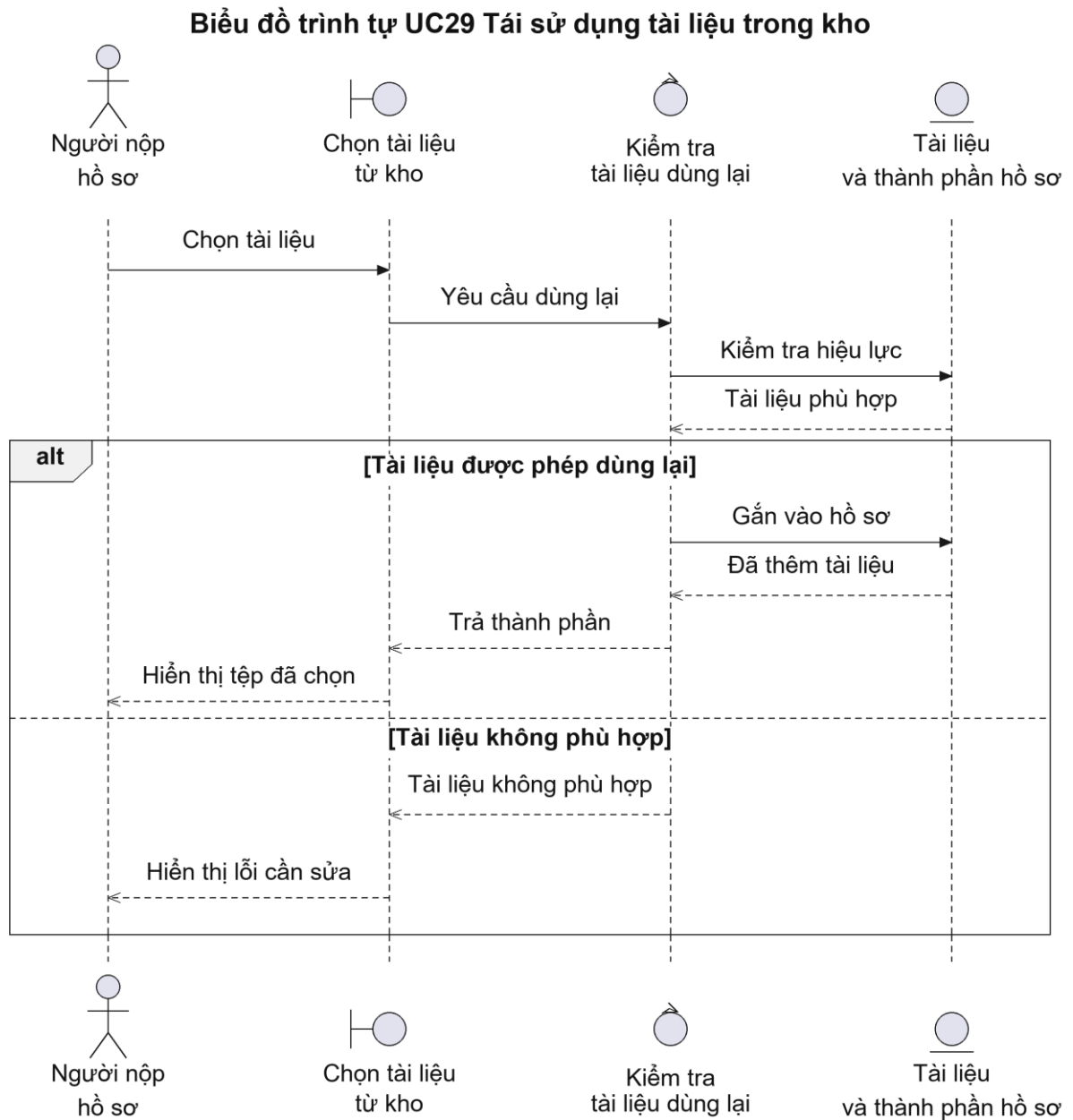
Hình 2.110: Biểu đồ trình tự của Use case UC29
